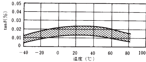
誘電正接-温度特性 (at 1kHz)
